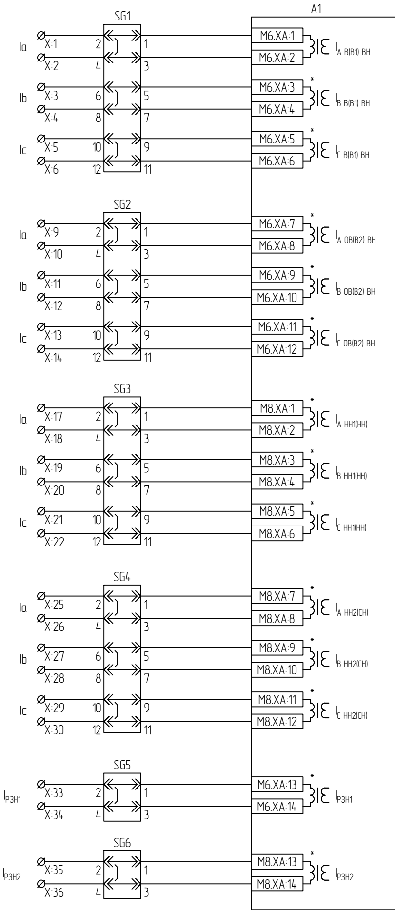
Цепи переменного тока А1
