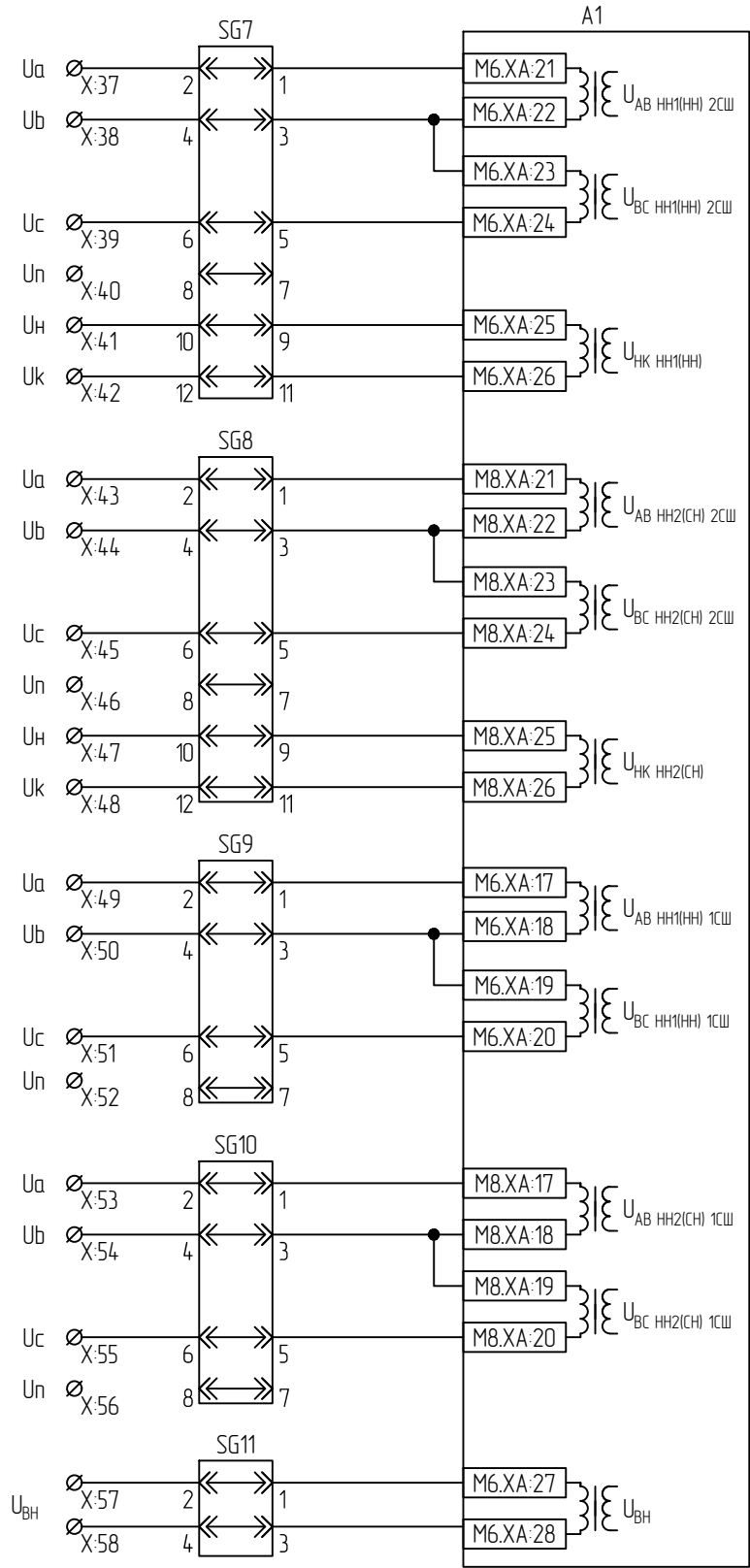
Цепи переменного и напряжения А1
